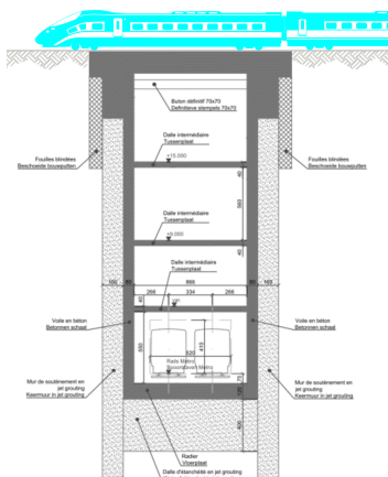
Schéma présentant l'infrastructure M3© Beliris
