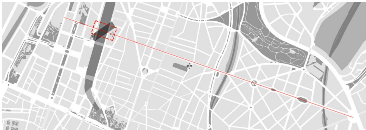
Plan présentant la rue et l'avenue Rogier ainsi que l'infrastructure M3 et la zone de percée © Google Maps
