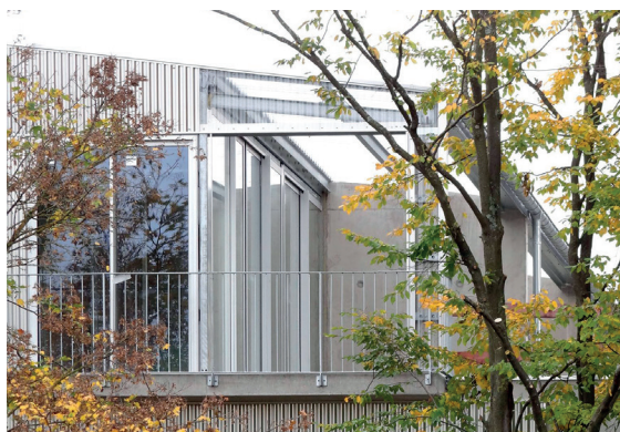
Extension par ajout d'une structure légère en toiture - Ballast Architecten. Uitbreiding door toevoeging van lichte structuur op het dak - Ballast Architecten.
