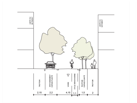
Rue Vandermeersch : suggestions Vandermeerschstraat: suggesties
