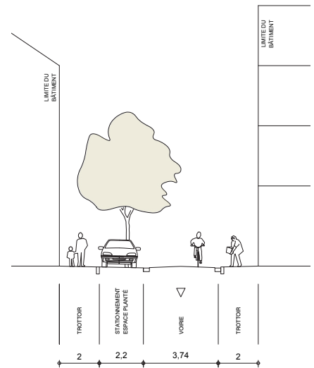
Rue Verte : suggestions Groenstraat (voor en na): suggesties
