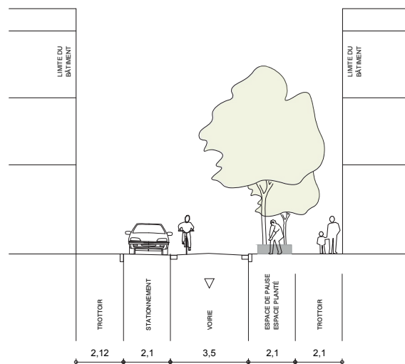
Rue Dupont : suggestions Dupontstraat: suggesties
