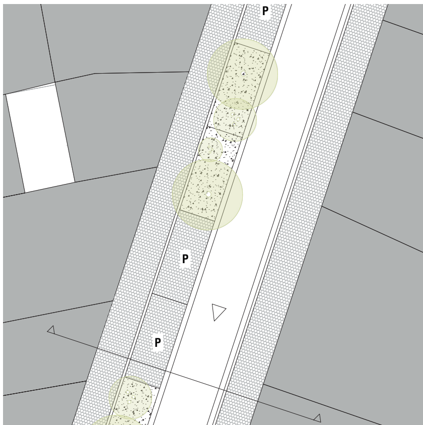
Rue de la Poste (plan à gauche) : suggestions.
